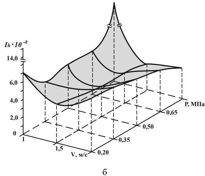
Рис. 3. Вплив питомого навантаження ( P ) і швидкості ковзання ( v ) на коефіцієнт тертя (а) і інтенсивність лінійного зношування (б) фенілону С-2
