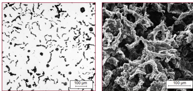
Рис.1. Мікроструктура чавуну з вермикулярним графітом [15].
