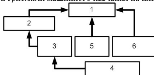
Рис. 1. Комплексна діагностика автомобільних двигунів на стисненому повітрі: 1 – Експертна система; 2 – Телекомунікаційні засоби зв'язку 3 – Бортова система діагностики 4 – Діагностика гальмівної системи 5 – Стендова діагностика 6 – Дорожні випробовування
