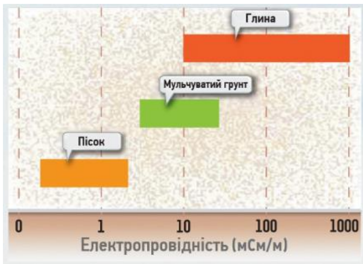
Рис. 1 – Електропровідність ґрунту
