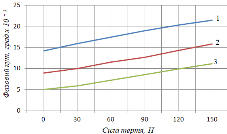
Рисунок 3. Вплив сухого тертя на параметр «фазовий кут» за різних значень коефіцієнта демпфірування амортизатора
