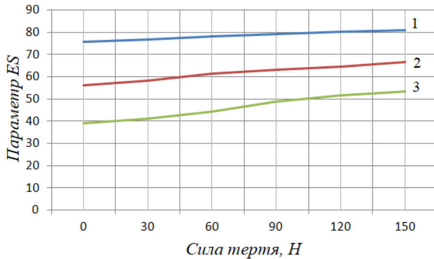
Рисунок 2. Вплив сухого тертя на «параметр EuSAMA» при різних значеннях коефіцієнта демпфірування амортизатора
