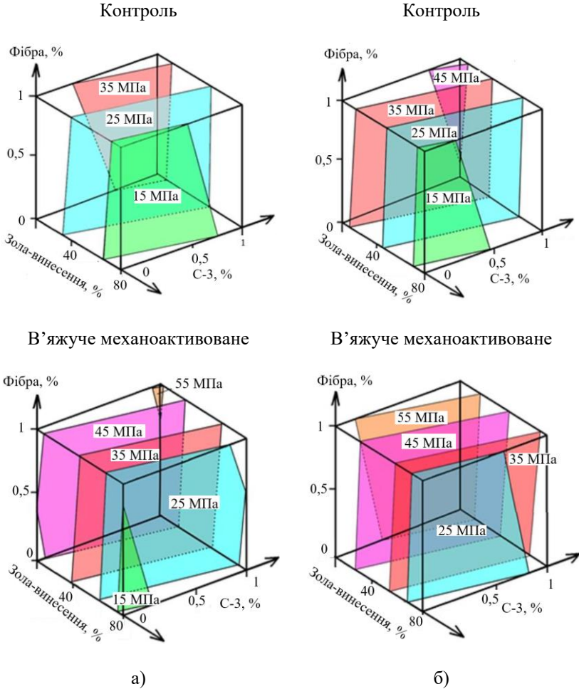
Рисунок 1. Вплив механоактивації на міцність бетону f_{cube} : а – 7-а доба твердіння; б – 28-а доба твердіння
